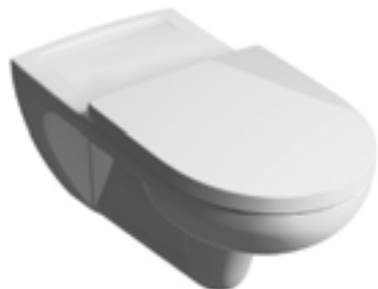
WAND-WC aus Sanitärkeramik, mit Spülrand, mit PflegePLUS, Breite: 355 mm, Tiefe: 700 mm
