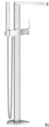
EINHAND-WANNENBATTERIE verchromt, Höhe: 901 – 1.005 mm, Ausladung: 282 mm
